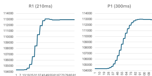
Figura 19 - Resposta Filtros R1 e P1
