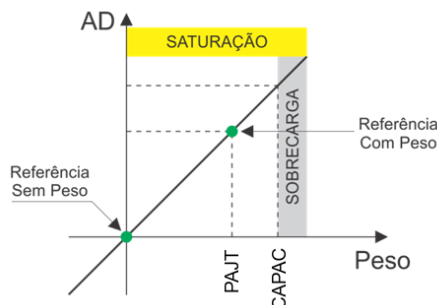
Figura 67 - Curva de Ajuste
