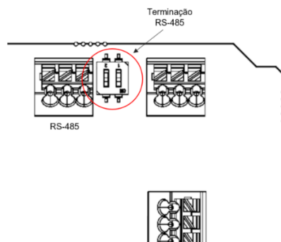
Figura 31 – Chaves de acionamento do terminador (no destaque). Indicador Linha 3100D, necessário abrir a caixa para ter acesso.
