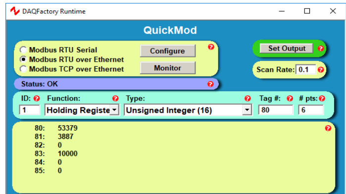
Figura 22 – Leitura de peso e status do indicador via Modbus-RTU over Ethernet Solução de problemas comuns:
