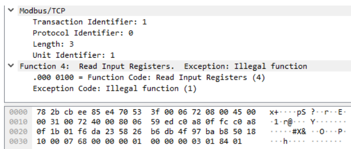
Figura 24 – Software Wireshark, mensagem função inexistente
