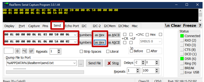
Figura 28 – Comando de leitura de peso e status, comando remoto de tara via RealTerm
