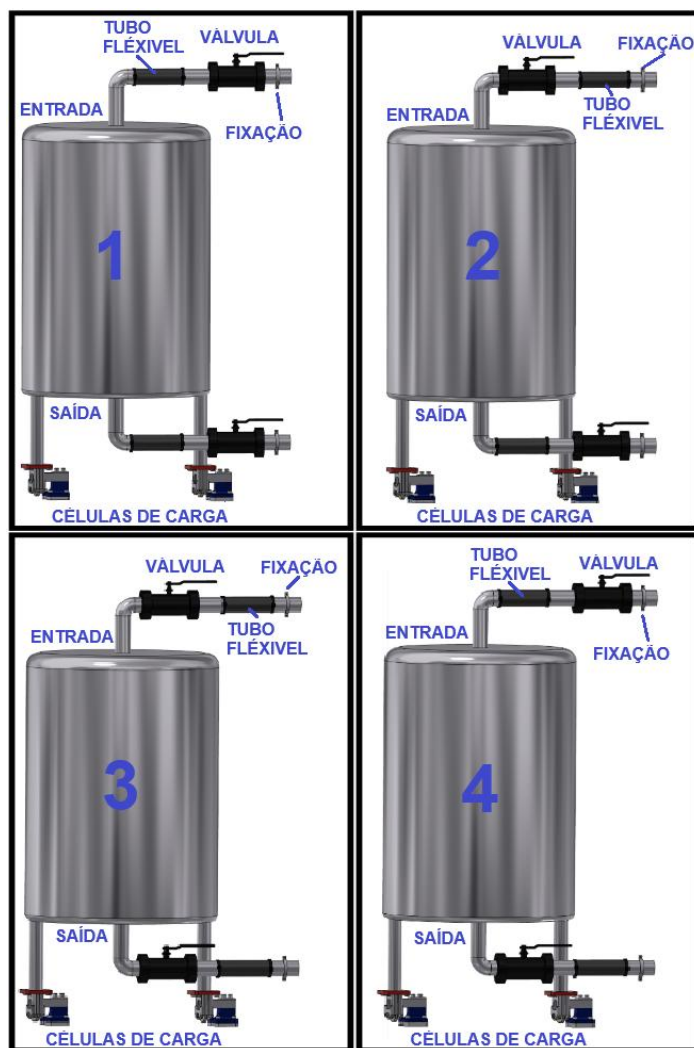
Figura 72 - Exemplo de Aplicação – Tanque
