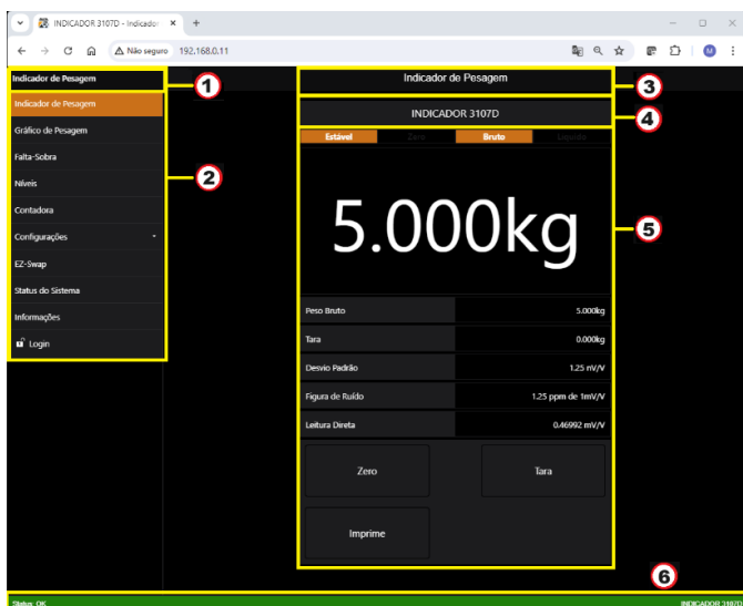
Figura 48 – Estrutura página inicial Alfa Web Monitor
