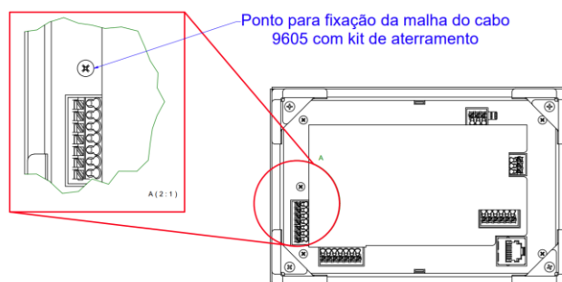
Figura 3 – Linha 3100DS detalhe local fixação terra
