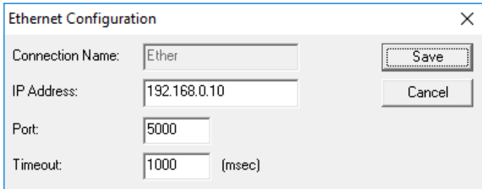
Figura 21 – Configuração no software DAQFactory. Deve-se colocar o IP e porta locais configuradas no indicador
