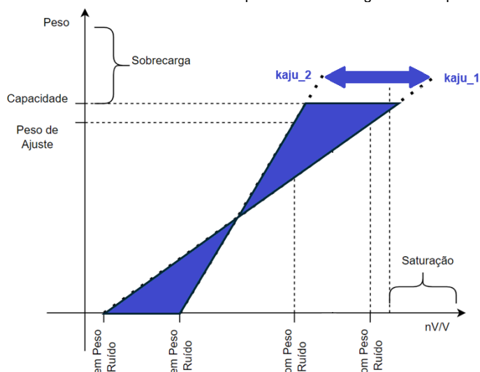
Figura 70 - Influência Peso Ajuste - Exemplo 1
