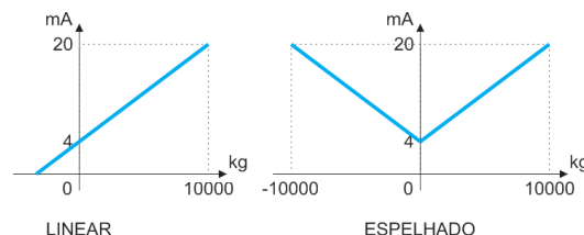
Figura 42 – Comportamento da Saída Analógica (LINEAR e ESPELHADO)
