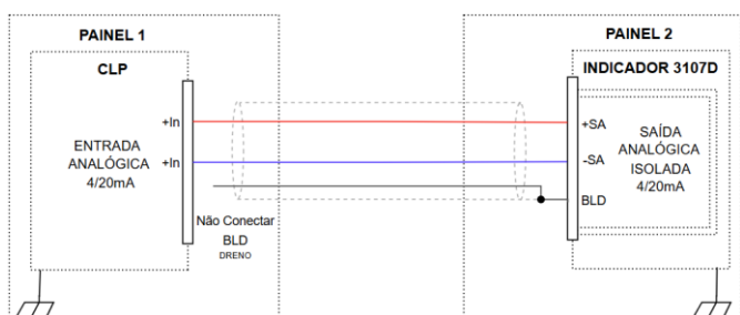
Figura 41 - Conexão do loop de corrente 4/20mA
