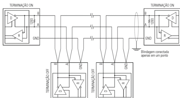
Figura 32 – Exemplo de esquema para linha de comunicação RS485 com utilização correta de terminadores
