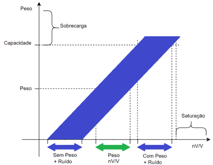
Figura 68 - Capturas de Peso - Exemplo 1
