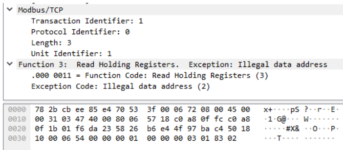
Figura 25 – Software Wireshark, mensagem de registrador inicial de leitura e/ou escrita e/ou quantidade de registradores inexistentes
