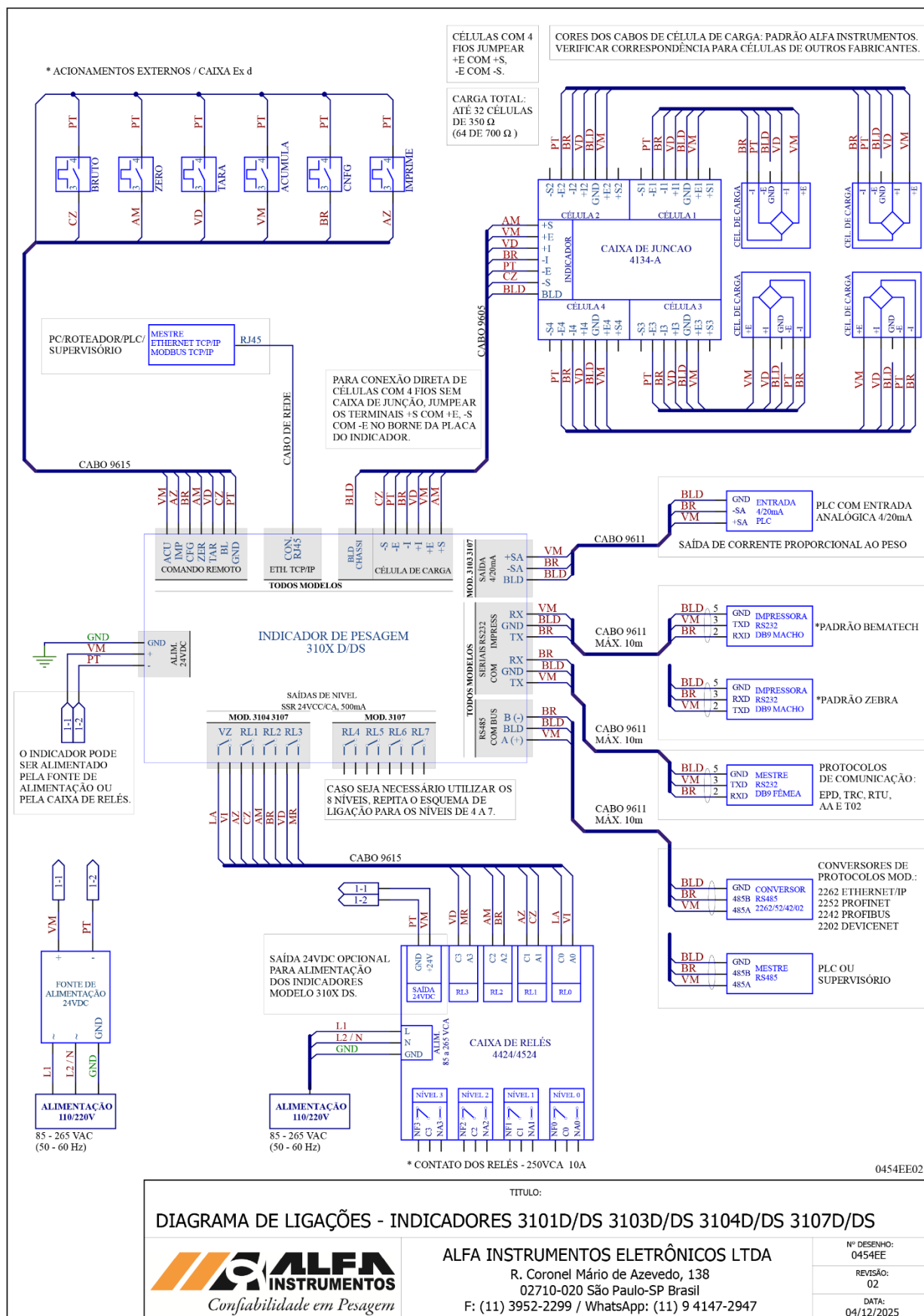
Figura 17 – Diagrama de conexões elétricas da família 3100D/DS
