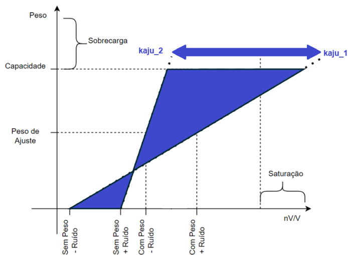
Figura 71 - Influência do Peso de Ajuste - Exemplo 2
