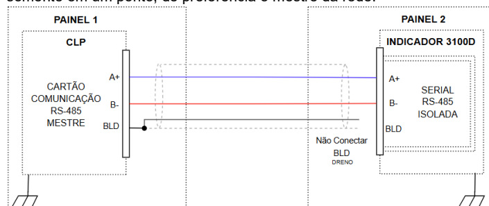
Figura 34 – Conexão da Blindagem RS-485
