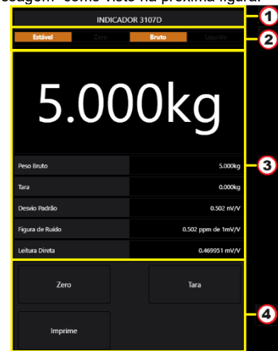
Figura 49 – Página Indicador de Pesagem via Alfa Web Monitor
