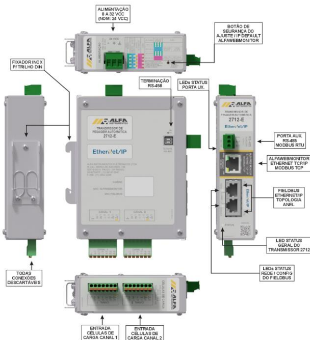
Figura 1 – Transmissor de Pesagem Automática 2712
