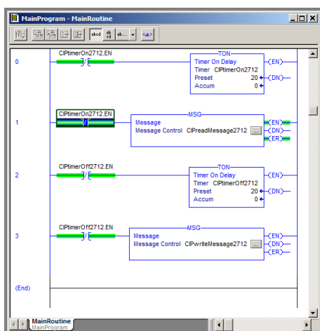
Figura 86 – Estrutura do programa no RSLogix 5000
