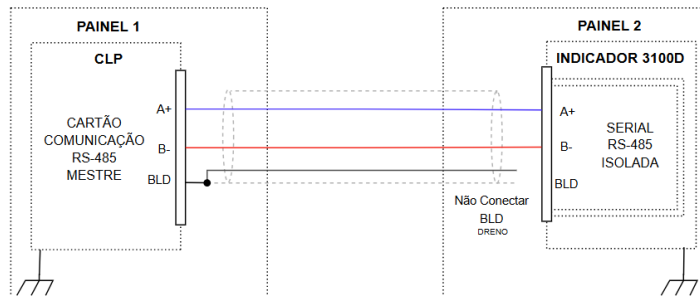
Figura 38 – Conexão da Blindagem RS-485
