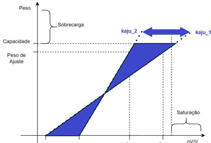
Figura 50 – Influência Peso Ajuste - Exemplo 1
