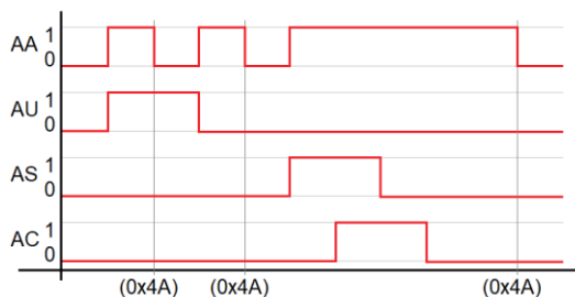
Figura 166 – Comportamento do acionamento do bit AA (Alteração do Alarme)
