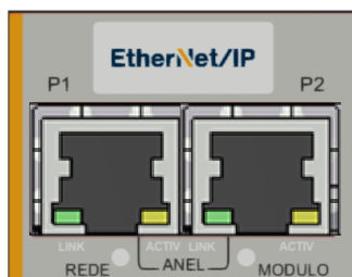
Figura 70 – Detalhe da posição dos leds de status da porta EtherNet/IP™
