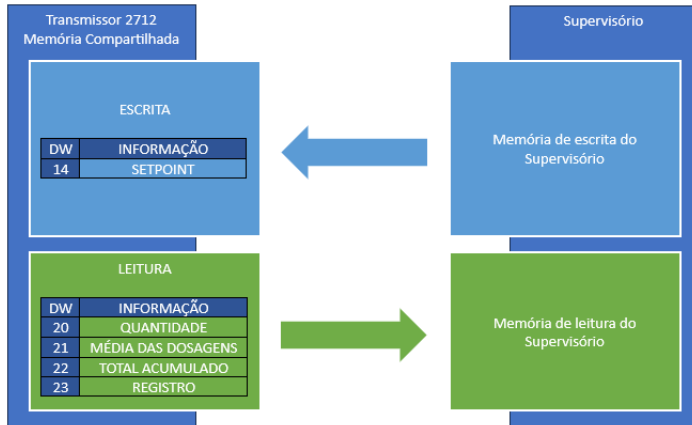
Figura 162 – Exemplo da troca de dados do Supervisório configurado com FIXED e acesso a Memória Compartilhada
