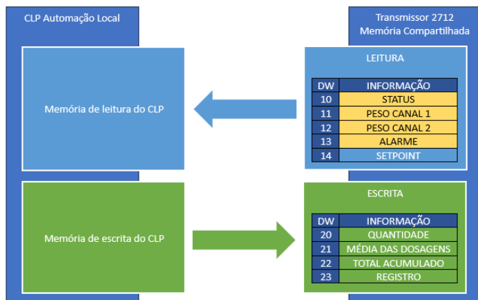
Figura 157 – Exemplo da troca de dados do CLP configurado com PGM e acesso a Memória Compartilhada
