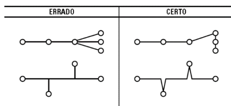
Figura 37 – Exemplo de geometria da rede
