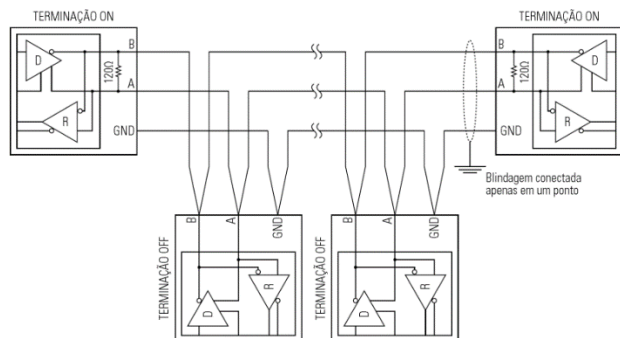
Figura 36 – Exemplo de esquema para linha de comunicação RS485 com utilização correta de terminadores
