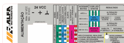
Figura 2 - Posição Botão de Ajuste
