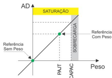
Figura 47 – Curva de Ajuste
