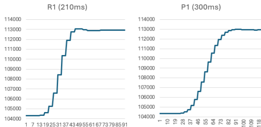
Figura 28 - Resposta Filtros R1 e P1
