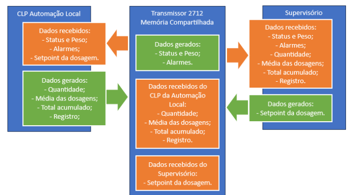
Figura 155 – Exemplo da troca de dados entre as portas de comunicação utilizando a Memória Compartilhada do Transmissor 2712
