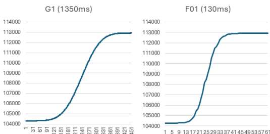
Figura 29 - Resposta Filtros G1 e F01
