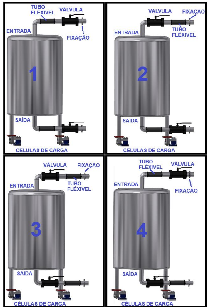
Figura 52 – Exemplo de Aplicação – Tanque
