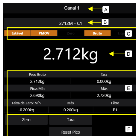
Figura 18 – Tela Indicador de Pesagem
