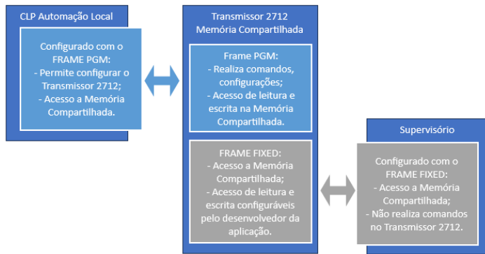
Figura 156 – Exemplo de uso das portas de comunicação com a Memória Compartilhada.
