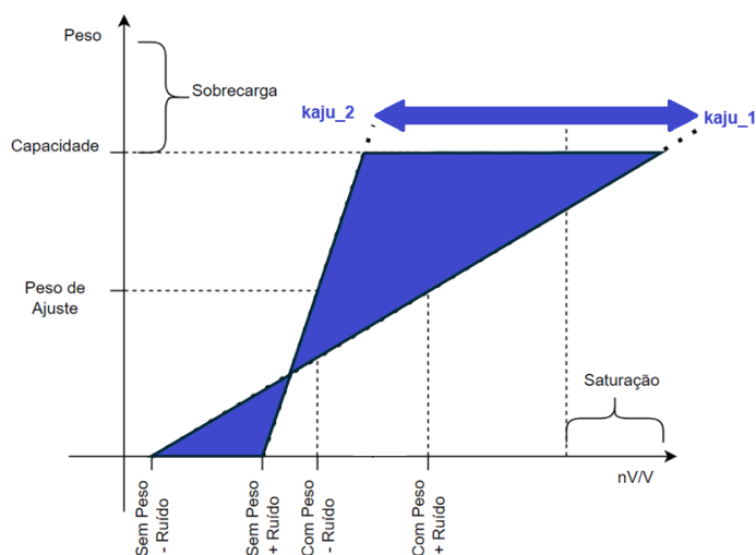
Figura 51 – Influência do Peso de Ajuste - Exemplo 2
