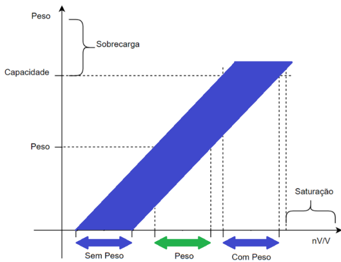
Figura 48 – Capturas de Peso - Exemplo 1
